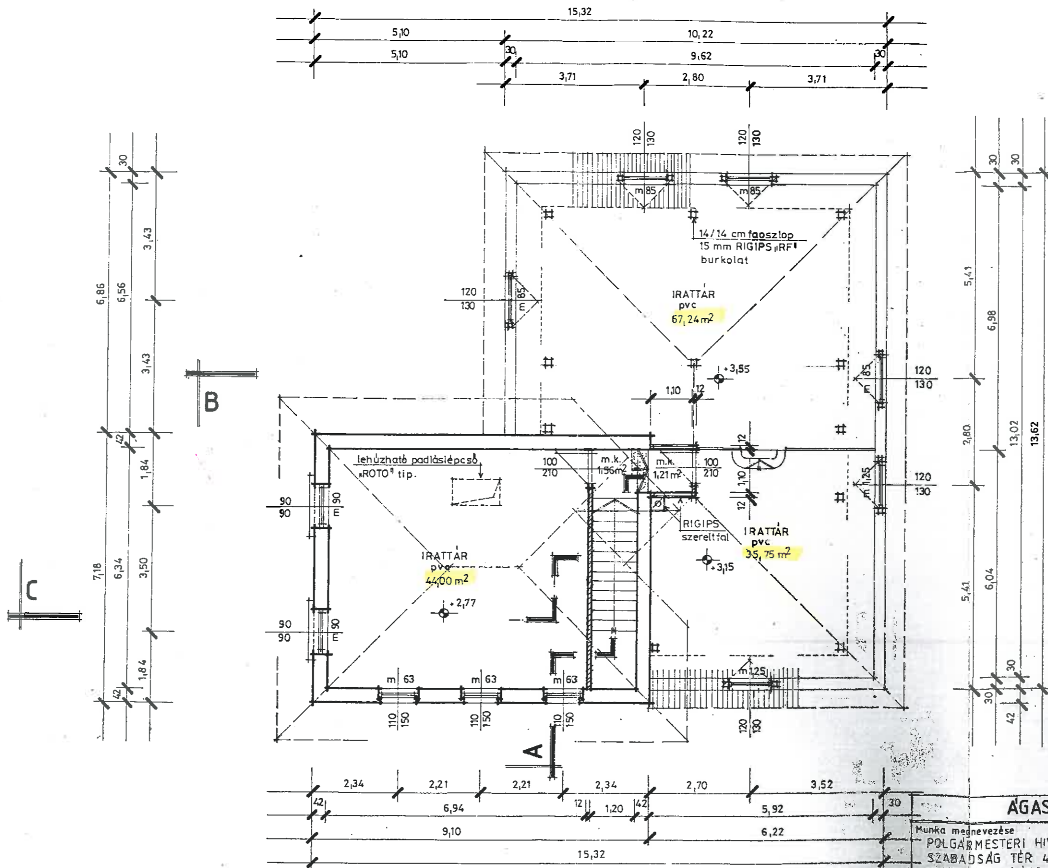
TETŐTÉRI ALAPRAJZ m 1:100
