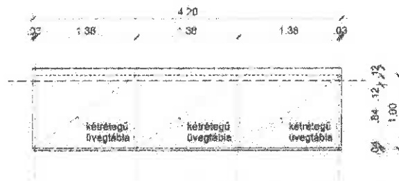
FELÜLNÉZET
