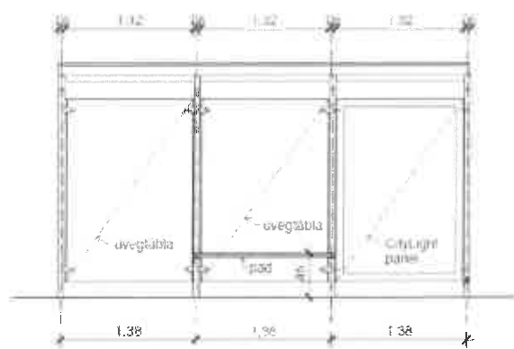
ELÖLNÉZET
