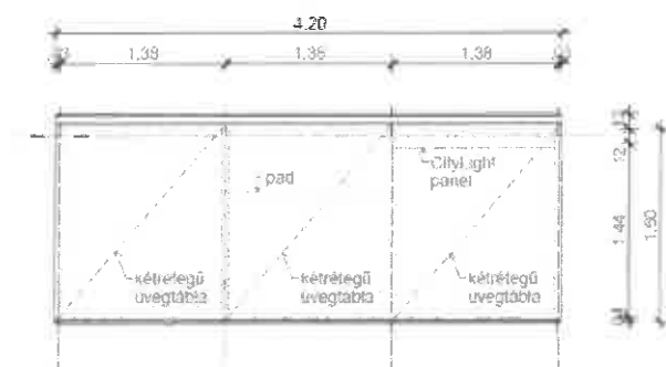
FELÜLNÉZET
