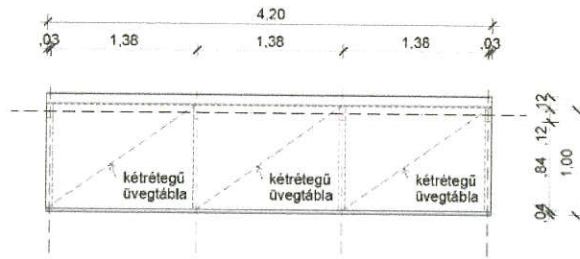
FELÜLNÉZET
