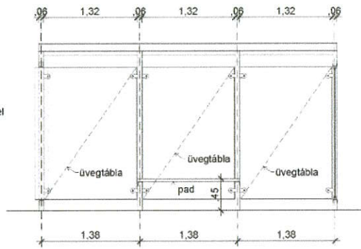
ELŐLNÉZET
