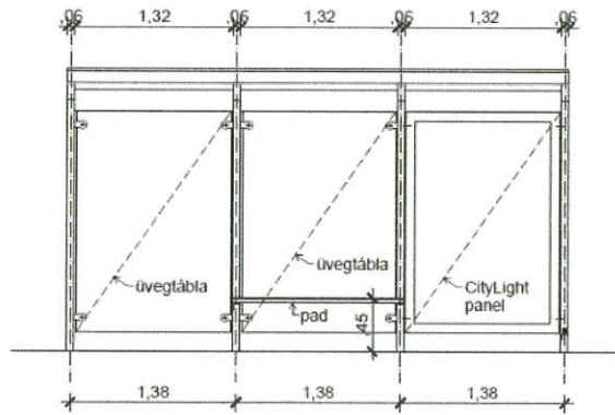
ELŐLNÉZET
