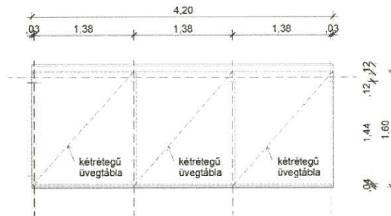
FELÜLNÉZET
