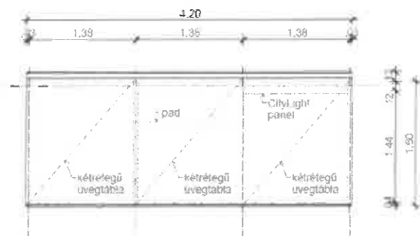
FELÜLNÉZET
