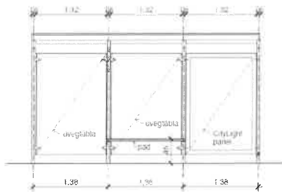
ELÖLNÉZET
